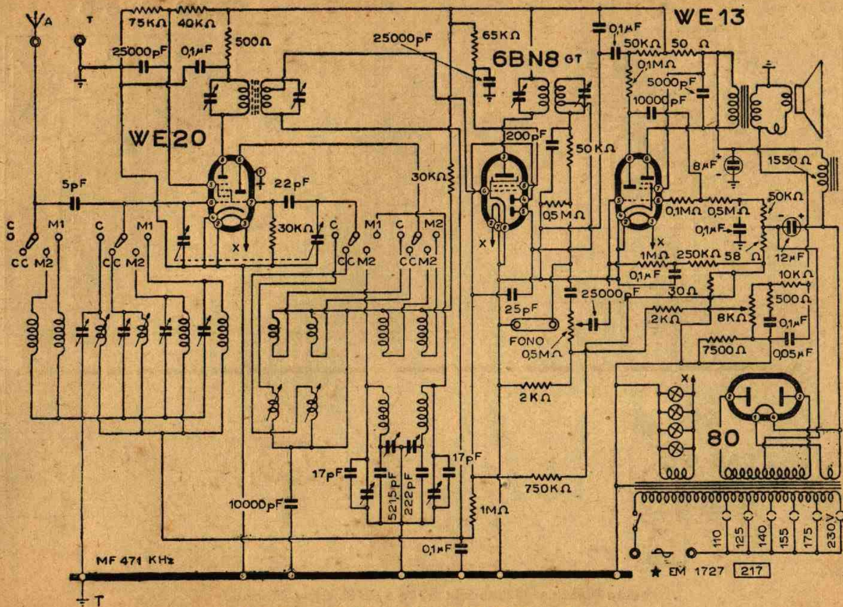
Lo schema elettrico del mod. S 41 Magnadyne.
